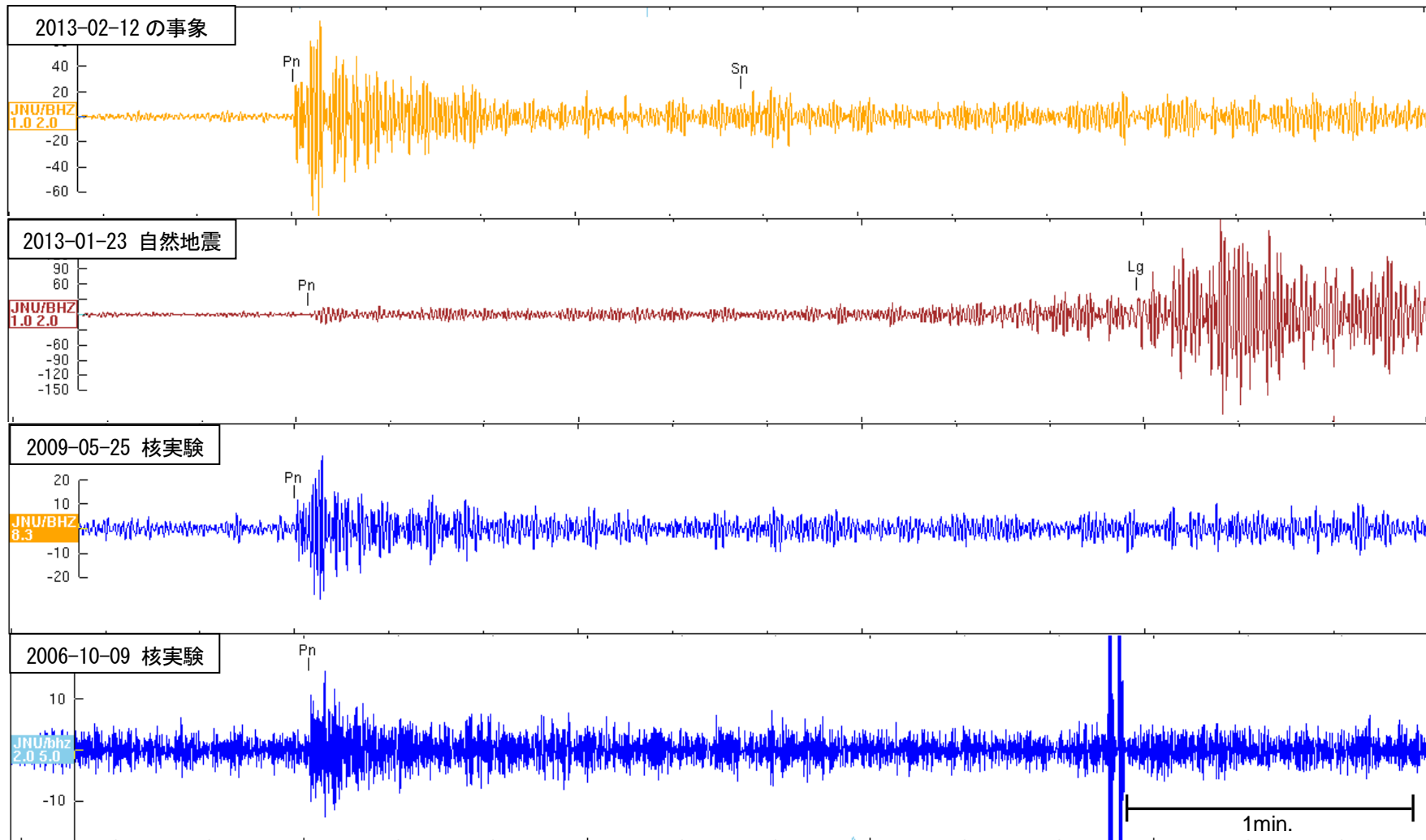
JNU (大分県日田市中津江) 観測点における観測波形の比較
