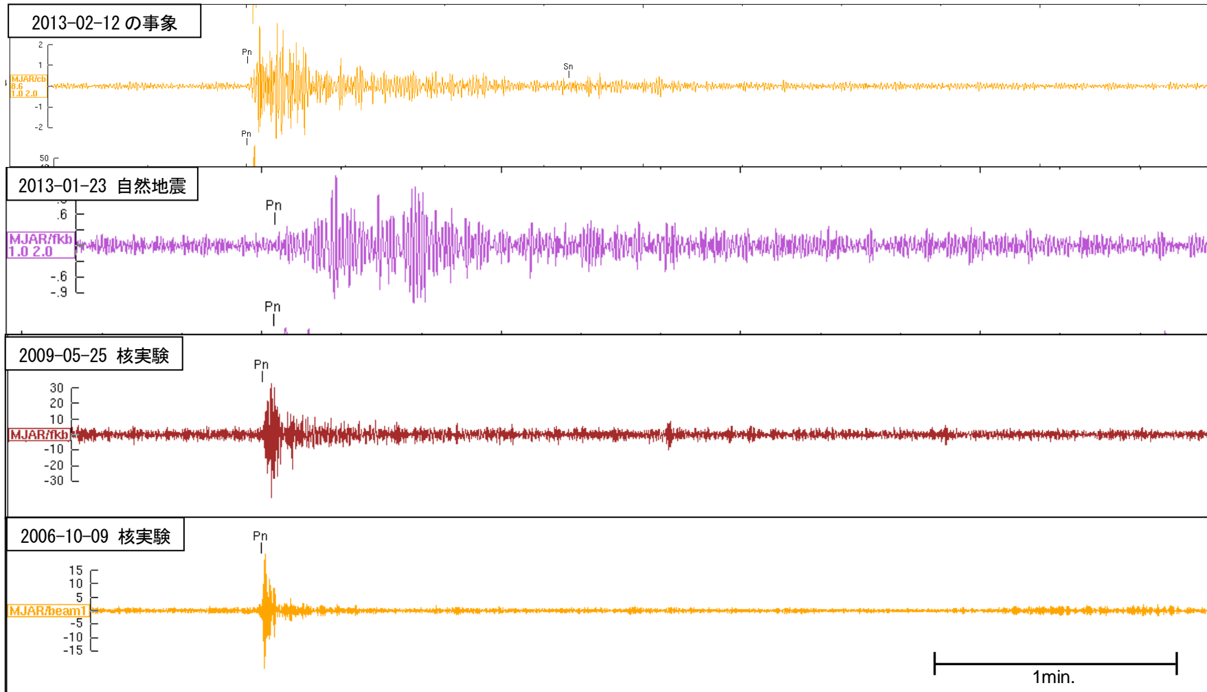
MJAR(長野県長野市松代)観測点における観測波形の比較
