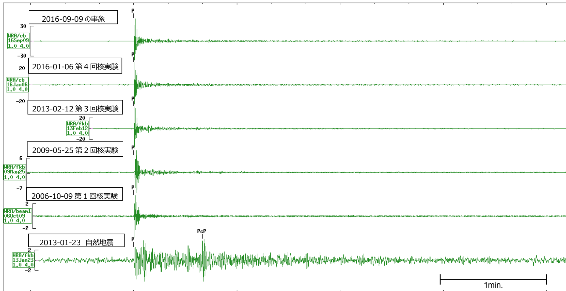
WRA（オーストラリア・ワラムガ）観測点における観測波形の比較（震央距離 6,800km、バンドパスフィルタ帯域：1.0～4.0Hz）
